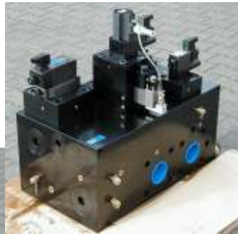
Ventilblöcke Manifolds
