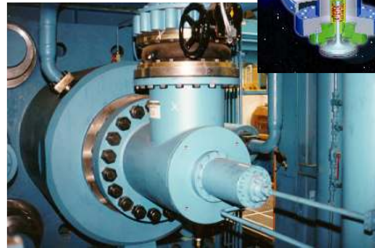
Füllventil Prefill valve
